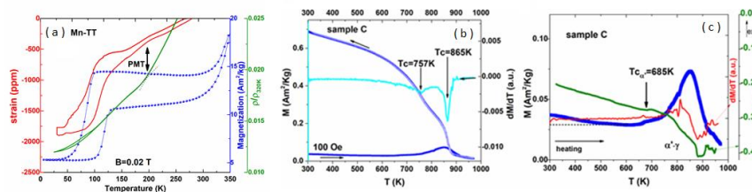
Fig. 3 Măsurători termomagnetice, termorezistive și de expansiune termică liniară ale probei \text{Ni}_{50}\text{Mn}_{20}\text{Ga}_{27}\text{Cu}_3 tratate pentru 20 min la 400°C (a). Curbele termomagnetice la temperaturi înalte (b) și comportamentul magnetic din scanarea DSC și dM/dT pe curba de încălzire (c) pentru proba \text{Fe}_{57}\text{Mn}_{27}\text{Si}_{11}\text{Cr}_5 .
