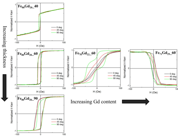
Fig. 2 Curbele de magnetizare MOKE ale filmelor amorfe Fe-Gd la unghiurile azimutale 0°, 45°, și 90°.
