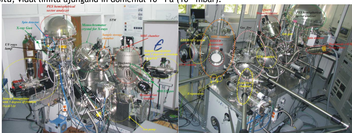
Figura 1. Fotografie și desemnarea principalelor elemente componente ale clusterului de știința suprafețelor, format din instalațiile de epitaxie din fascicul molecular, microscopie de baleiaj cu efect tunel și instalația de spectroscopie de fotoelectroni cu rezoluție unghiulară și de spin. Acest cluster a primit denumirea CoSMoS (Combined Spectroscopy and Microscopy on a Synchrotron) atunci când a fost conectat la linia de fascicul SuperESCA de la facilitatea de radiație de sincrotron Elettra, Trieste. Fabricant: Specs, Berlin, Germania.
