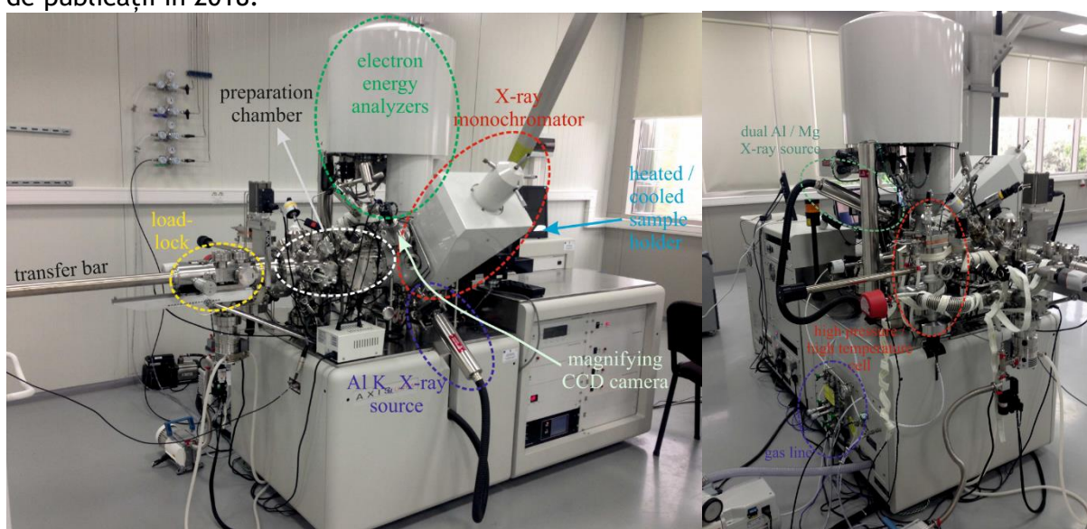
Figura 7. Instalația de spectroscopie de fotoelectroni cu posibilități de analiză pe arie microscopică și dotată cu celula de tratare a probelor în condiții de presiune și temperatură ridicată (4 bar / 1000 °C). Fabricant: Kratos, Manchester, Marea Britanie.
