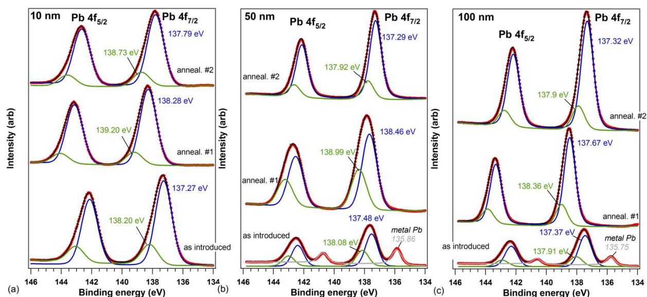
Figura 3. Spectre XPS ale Pb 4f măsurate pe straturi subțiri de 10 nm \text{Pb}(\text{Zr},\text{Ti})\text{O}_3(001) (a), 50 nm \text{Pb}(\text{Zr},\text{Ti})\text{O}_3(001) (b) și 100 nm \text{Pb}(\text{Zr},\text{Ti})\text{O}_3(001) (c) imediat după introducerea probei, după un prim tratament termic și după un al doilea tratament termic în atmosferă de oxigen. În cazul (a) s-a folosit
