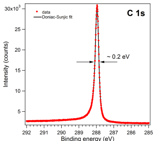
Figura 4. Spectru XPS al carbonului 1s măsurat pe un strat monoatomic de grafenă crescută pe un monocristal de Pt(001). Durata achiziției: 0,2 s/punct, 12 minute în total, cu un pas energetic foarte mic pentru XPS, 10 meV.
