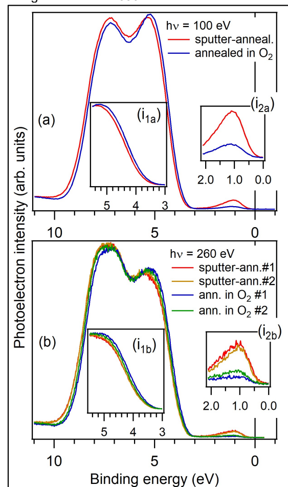
Figura 3. Spectre din banda de valență ale SrTiO 3 (001) după sputtering și în vid ultraînalt (curve roșii) și după tratament în oxigen ( 2 \times 10^{-7} hPa - 10^{-6} hPa, curbe albastre). Energia de excitare a fost 100 eV în (a) și 260 eV în (b); În (b), sunt prezentate spectre obținute imediat după preparare și după 5 ore de iradiere a probei cu fotoni în domeniul VUV (100
